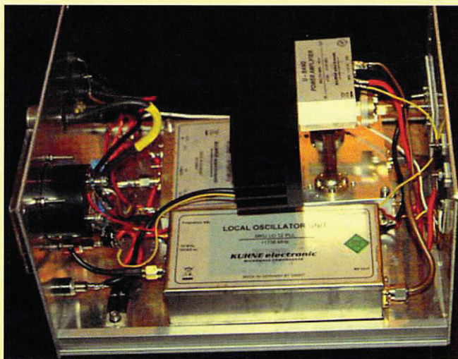
Bild 10: Blick in den 47 GHz-Transverter
