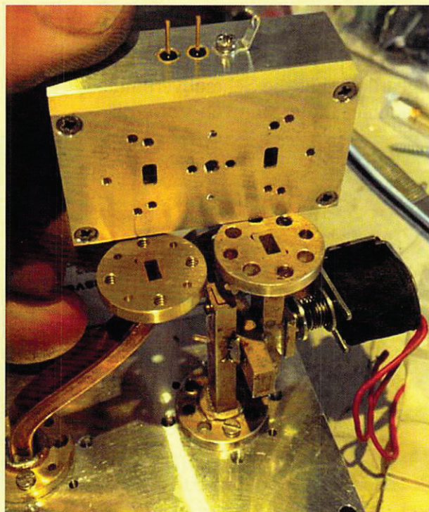
Bild 9: Montage 1 W Endstufe auf HL-Schalter
