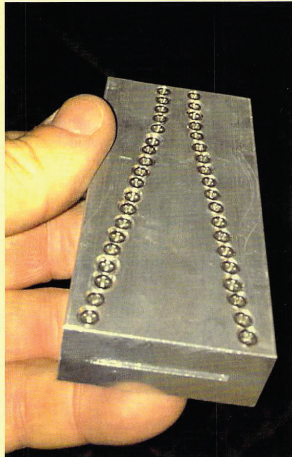
Bild 6: Sektorantenne für 47 GHz
