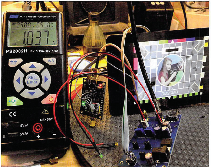
Abbildung 4: Der Testaufbau eines DATV-Senders mit dem Raspberry Pi, und der Mini-IQmod-Platine aus [1].
