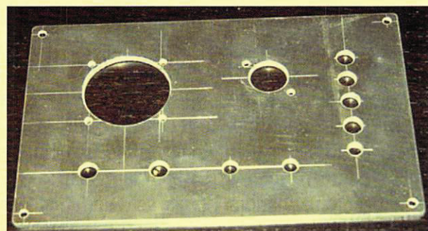
Bild 7: Entstehung Frontplatte
