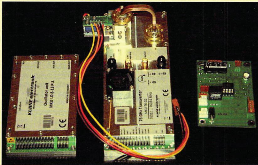
Bild 12: 76 GHz Komponenten mit montiertem Hohlleiterschalter
