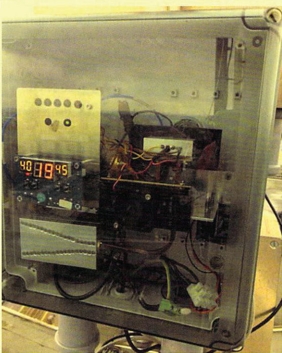
Bild 7: 47 GHz Bake
