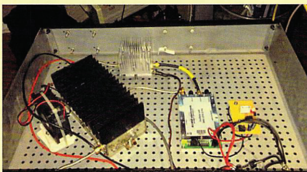
Bild 2: Innenleben der 9 cm Bake
