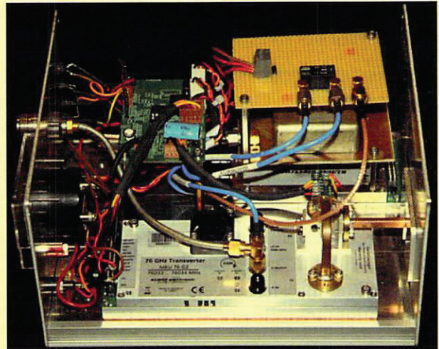
Bild 5: 76 GHz Transverter
