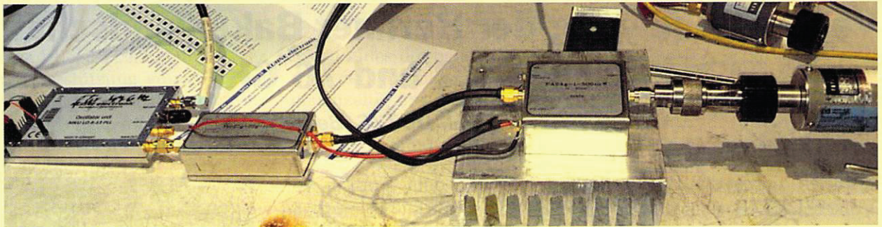
Bild 4: Probeaufbau 24 GHz-Bake
