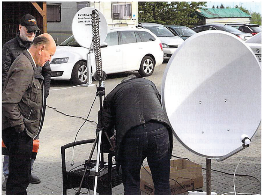
Abbildung 1: Für den Empfang des Satelliten QO-100 im 3-cm-Band kann eine handelsübliche Satellitenschüssel mit einem umgebauten LNB genutzt werden. Zum Senden benötigt man eine rechtsdrehend zirkular polarisierte Richtantenne für das 13-cm-Band.
